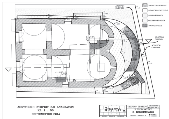
Εικ. 3. Κάτοψη του ναού και αποτύπωση των ανασκαφικών τομών.
