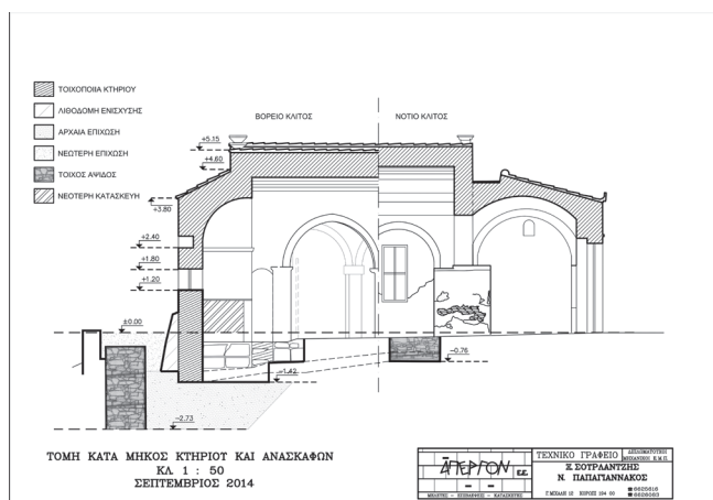
Εικ. 4. Κατά μήκος τομή ναού και ανασκαφικών ευρημάτων.
