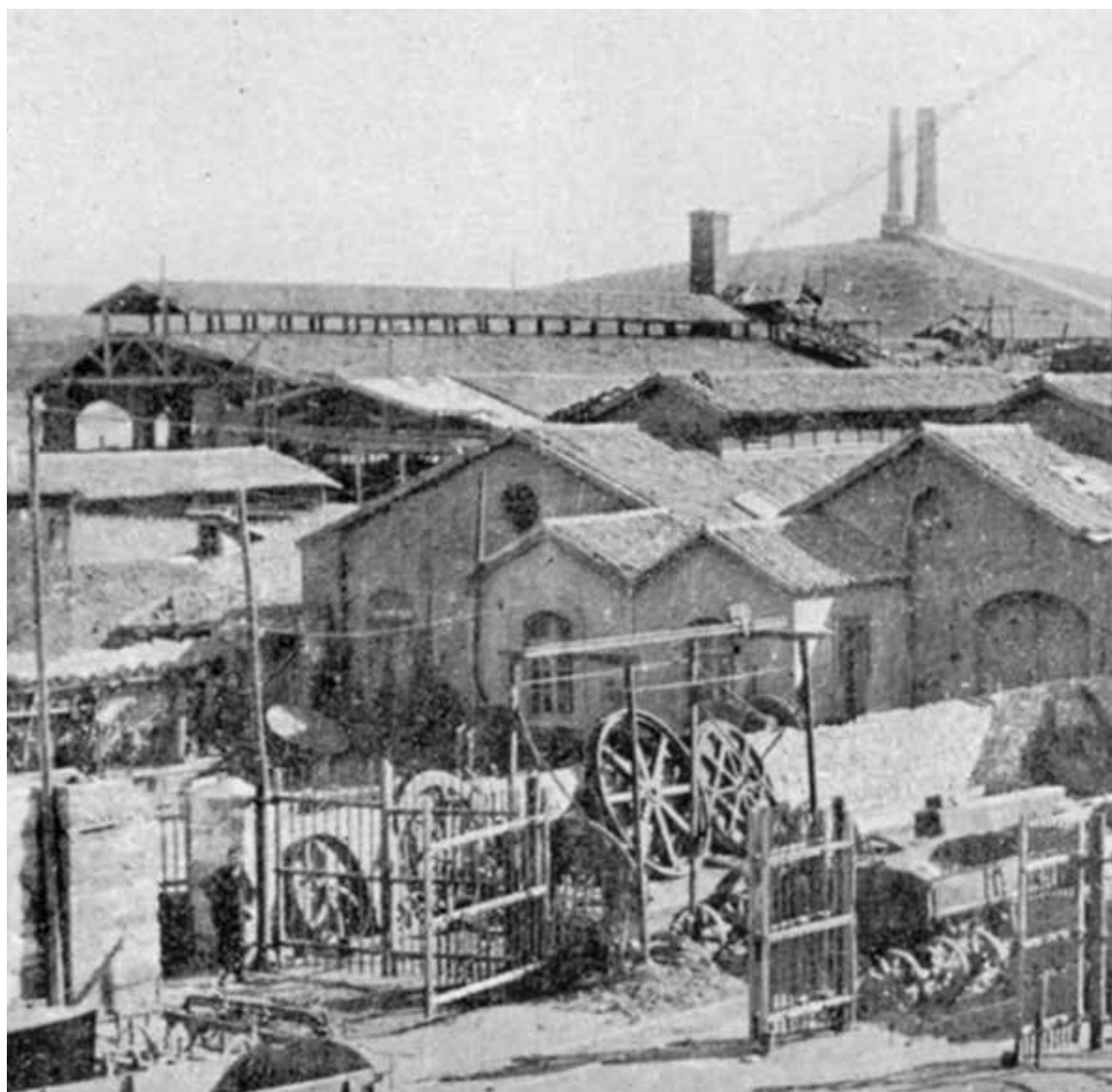
Το κτηριακό συγκρότημα του Μηχανουργείου και του Χυτηρίου (φωτ. 1911)
