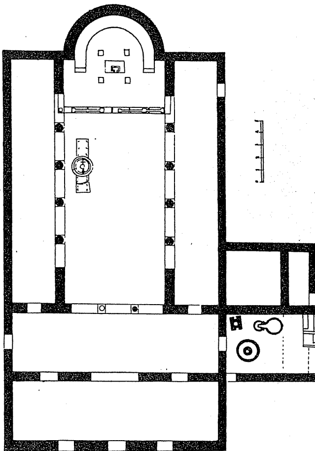
5. Βασιλική του Λαυρεωτικού Ολύμπου. Κάτοψη. (N. Κοτζιάς)
