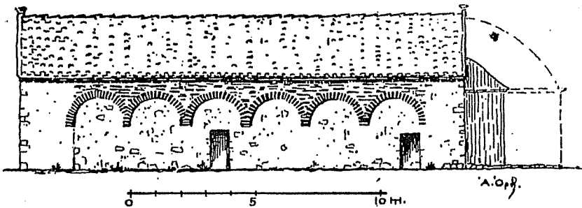
9. Βασιλική των Καλυβιών Κουβαρά. Άποψη του νοτίου τοίχου σχεδιασμένη από τον Α.Κ. Ορλάνδο
