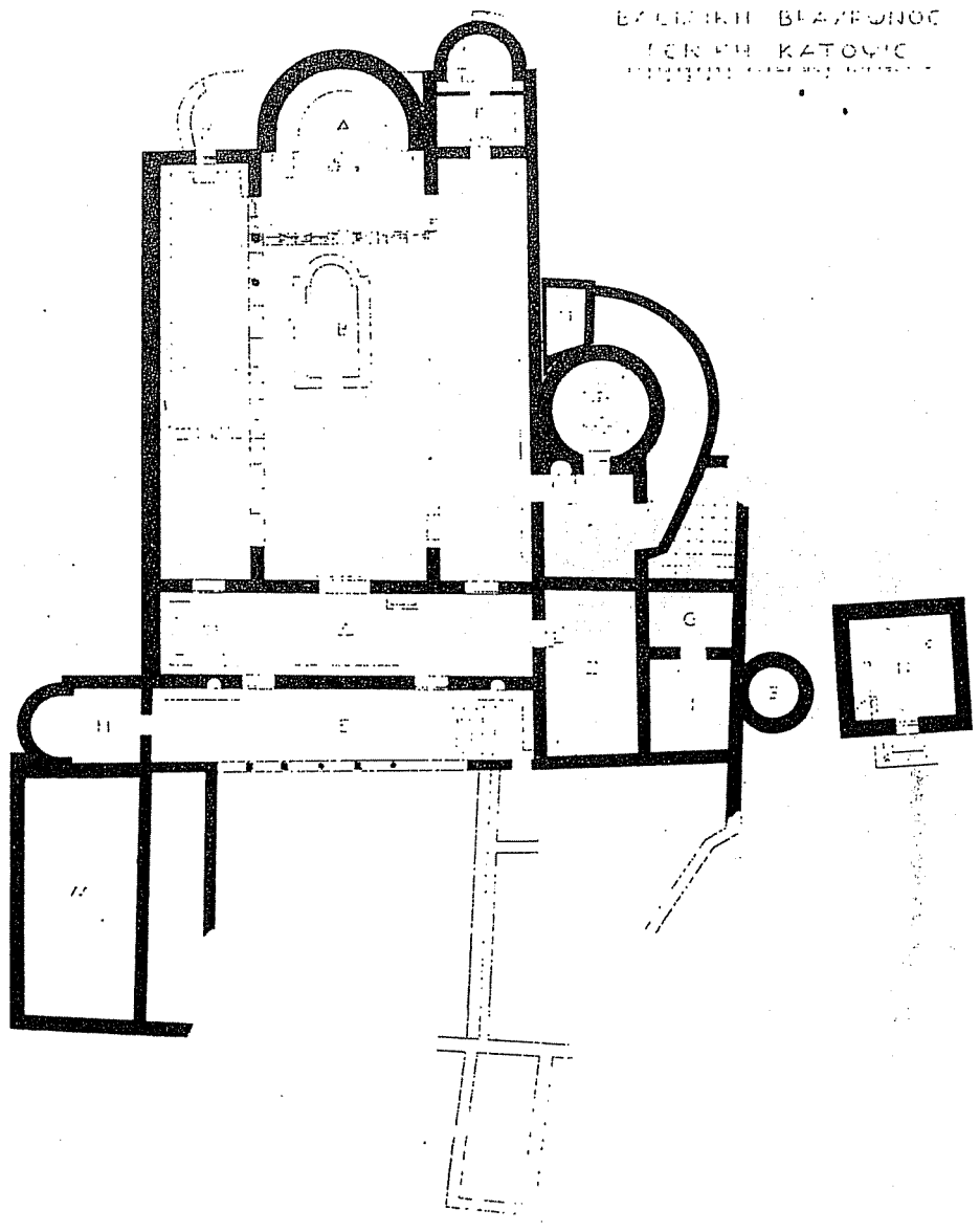
3. Βασιλική της ΒραΨώνας, Κάτοψη (Ε. Στίκας)
