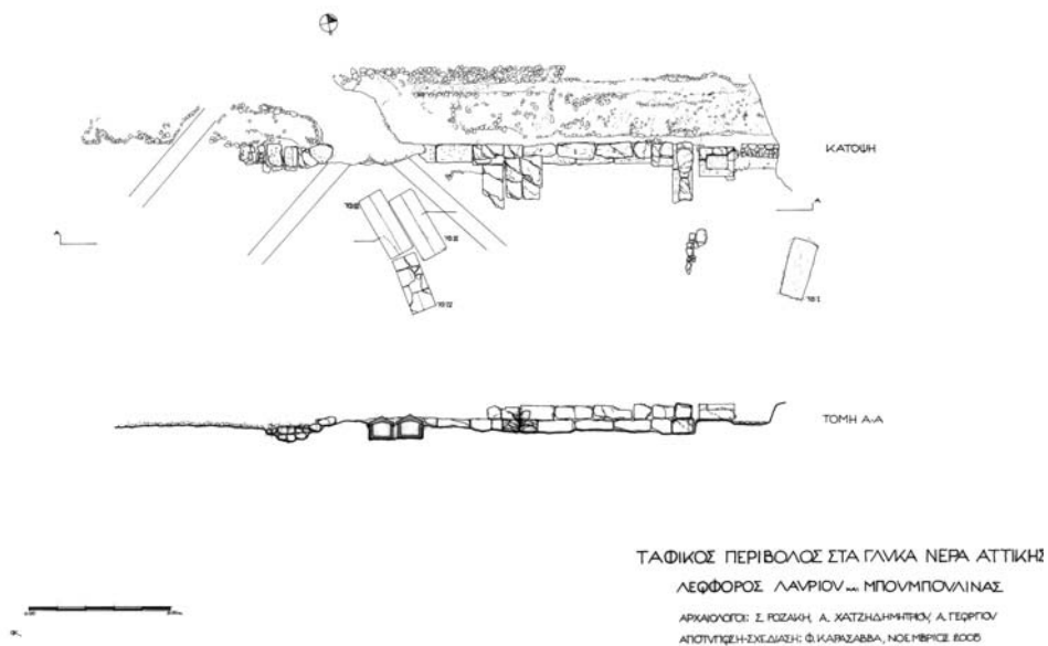
Εικ. 1. Γλυκά Νερά. Κάτοψη και Τομή του Ταφικού Περιβόλου.
