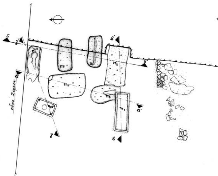
Σχ. 4. Κάτοψη ανασκαφής Οικοπέδου Κώτσια, Κλίμακα 1:50.
